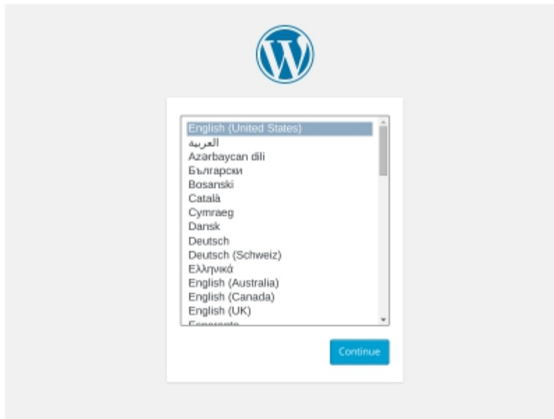
Fig. 7.11: WordPress instalação
